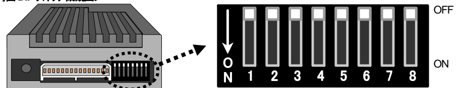
<背面 DIP スイッチ概観図>
