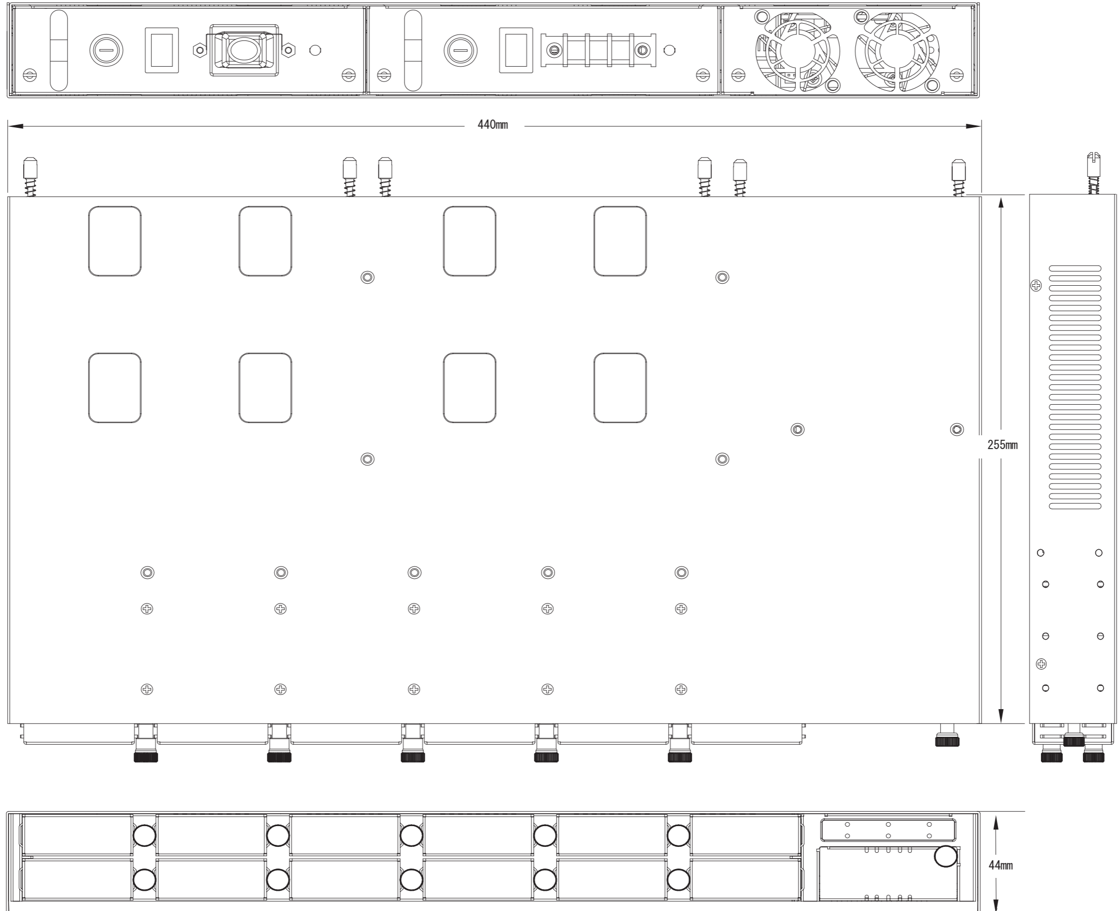
LEX1012外観図
