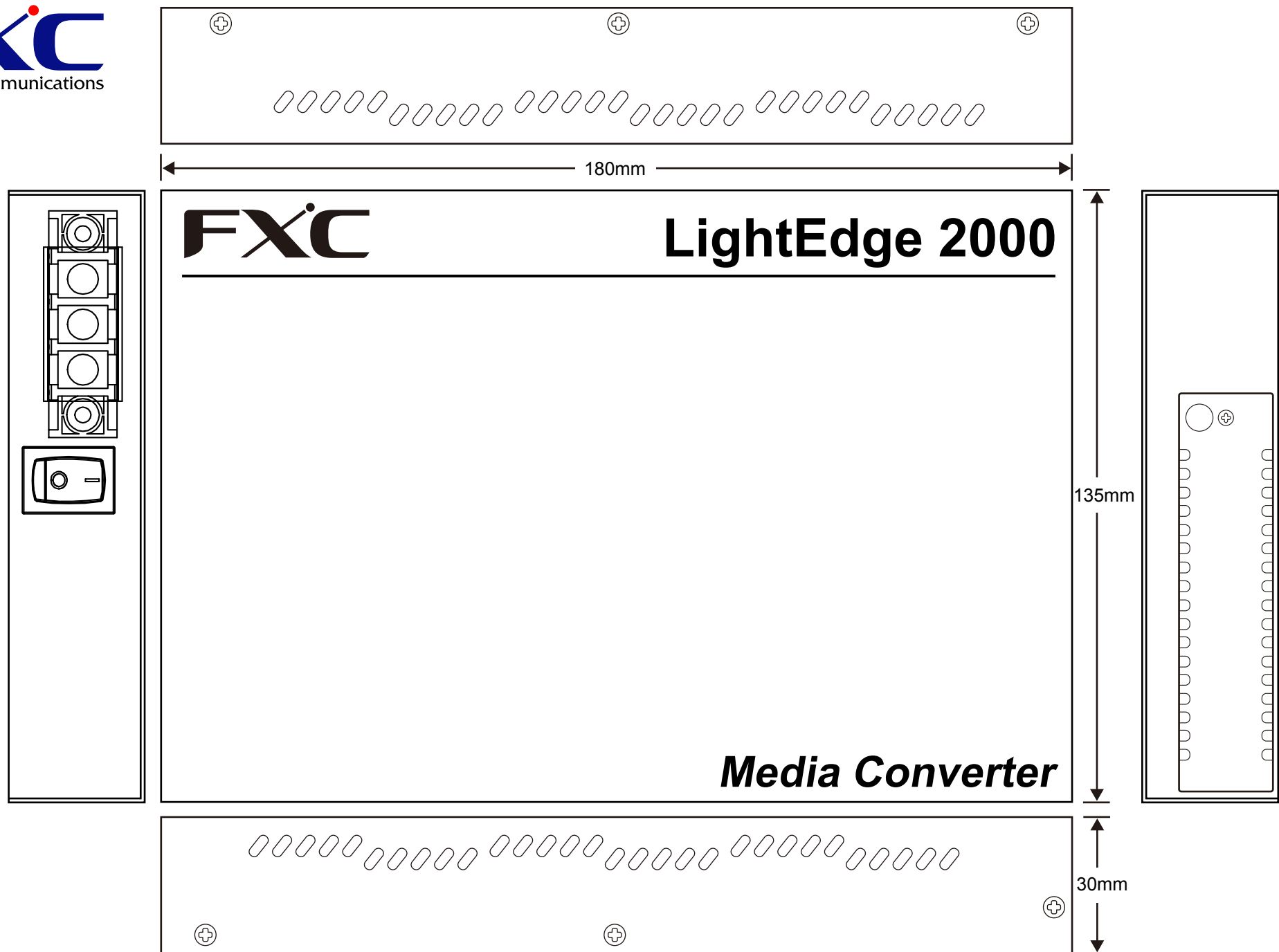
LE2001-45外觀圖
