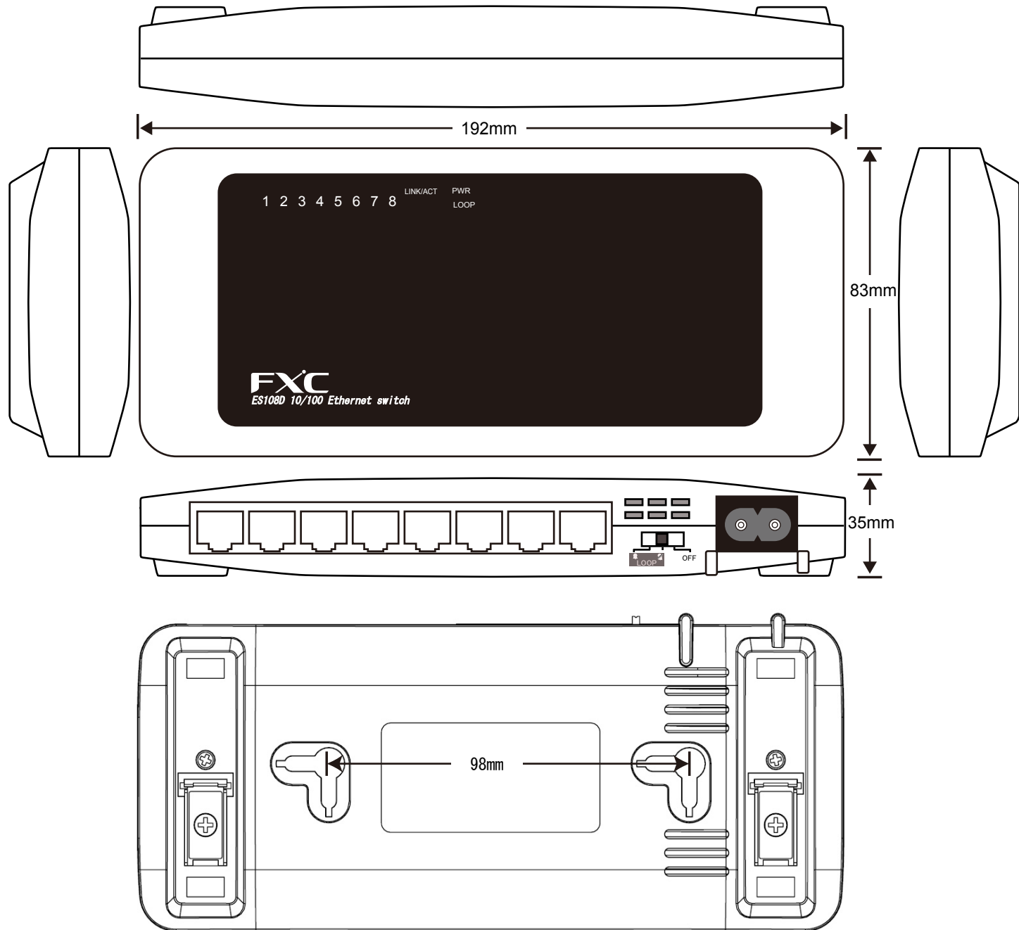
ES108D外観図
