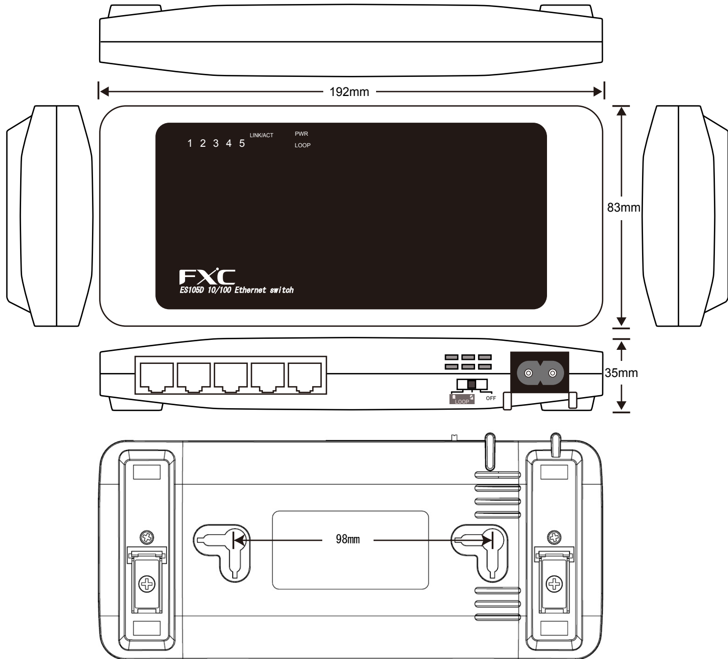
ES105D外観図
