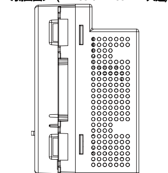
<側面図> (AE1031/AE1031PE 共通)
