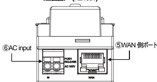
<上面図> (AE1031)
