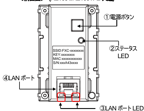
<前面図> (AE1031/AE1031PE 共通)
