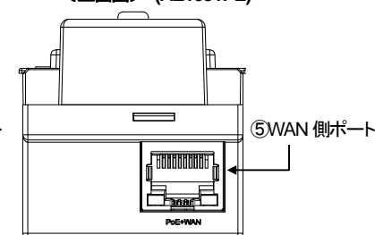
<上面図> (AE1031PE)
