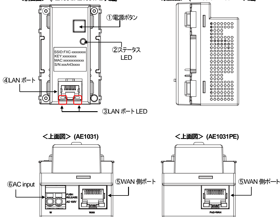
<前面図> (AE1031/AE1031PE 共通)
