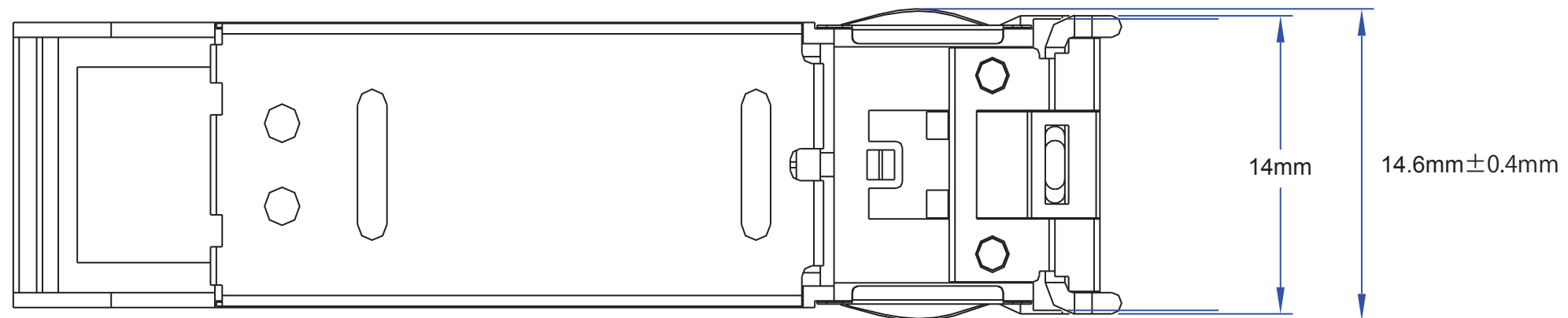
2芯LC TYPE2外觀図
